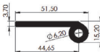
DOBRADIÇA 51,5 x 3,7
