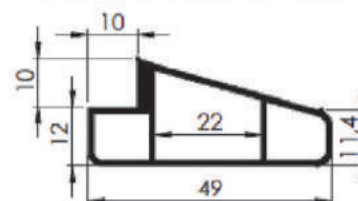
TUBO OBLONGO COM ABA 49 X 17 X 11,4
