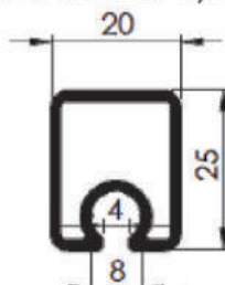
TRAVA TELA 25 X 20 X 1,5
