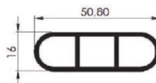
TRAVESSA 50,8 x 16 x 1,6
