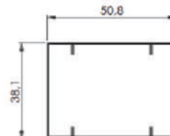
TUBO RETANGULAR (FRISO INTERNO) 50,8 X 38,1 X 0,95
