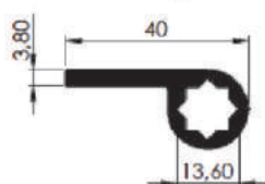
DOBRADIÇA FURO ESTRELA 40 x 3,8
