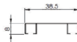
TRILHO INFERIOR GUIA ALTA
