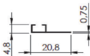
TRILHO INFERIOR MONO
