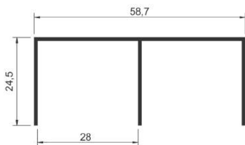
TM-001 Trilho superior 58,7 mm
