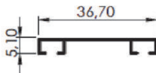
TRILHO INFERIOR MENOR
