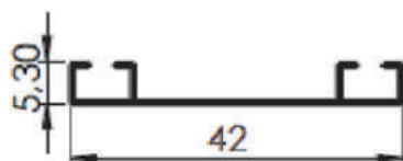
TRILHO INFERIOR MAIOR
