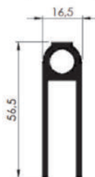
TRINCO 56,5 X 16,5
