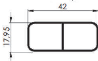
TRAVESSA BITUBULAR 42 X 18 X 1,3
