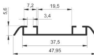
TM-004 Trilho inferior com aba 48 mm
