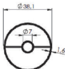
TUBO REDONDO 38,10 COM OLHAL
