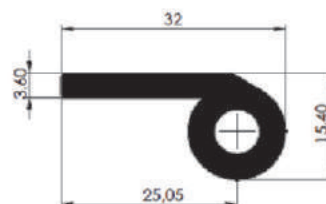
DOBRADIÇA 32 x 3,6
