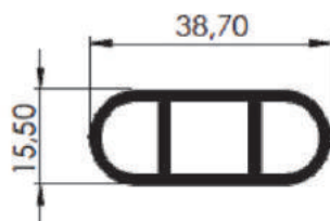
TRAVESSA 38,7 x 15,5 x 1,6
