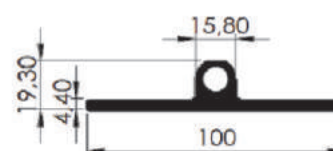
DOBRADIÇA 100 x 4,4
