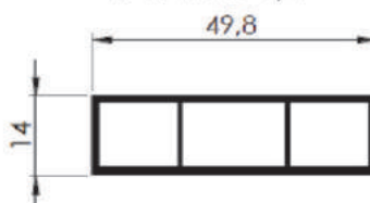
TRAVESSA TRITUBULAR 49 X 14 X 1,4
