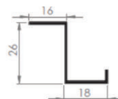
DESCANSO DE JANELA MAX AIR
