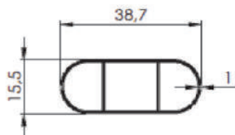
TRAVESSA 38,7 x 15,5 x 1,0
