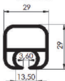
TRAVA TELA 29 X 29
