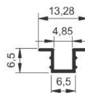
TM-010 Perfil "U" abas iguais 13 x 6,5 mm
