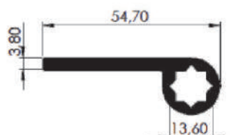
DOBRADIÇA FURO ESTRELA 55 x 3,8
