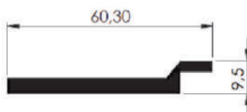
PLACA 60,3 X 9,5
